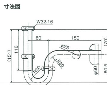
寸法図
