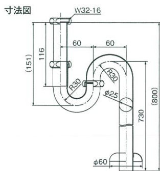
寸法図
