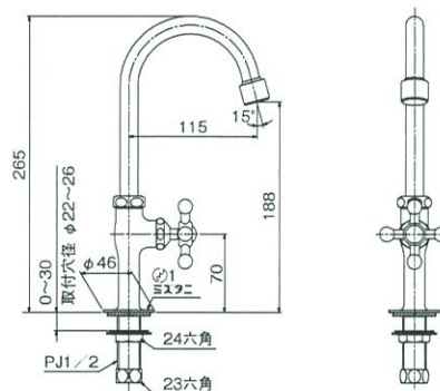
寸法図
