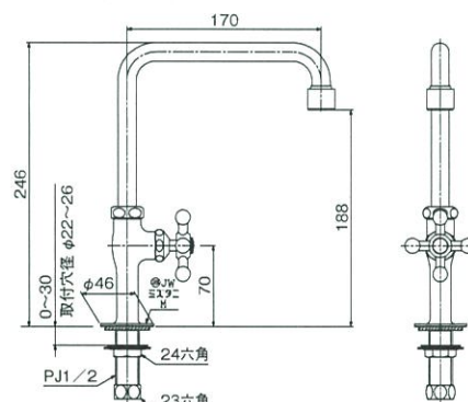
寸法図
